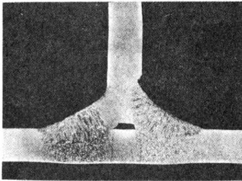
Şek. 201 — Yatay pozisyonda kaynak edilmiş T birleşmesinin, kaynak kenarında yanma çentiğini gösteren makro kesiti. Yavaş katılaşma tempolu rutil elektrod kullanılmıştır. (x2) (Baskıda % 50 küçültülmüştür).
